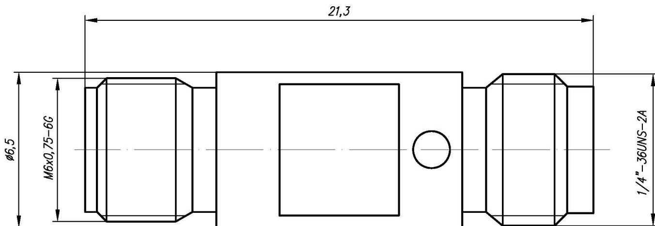
Рисунок коаксиального перехода
